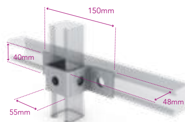
Deep Normal Top Hat Bracket
